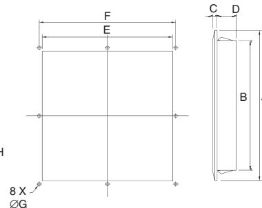
Фильтрующий вентилятор - RZF300
