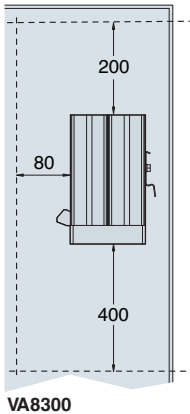
Минимальные монтажные расстояния
