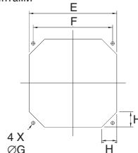
Фильтрующий вентилятор - RZF300
